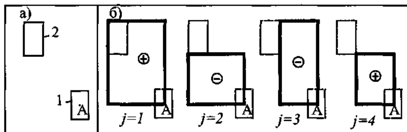
а - схема розташування фундаменту 1, що розраховується, і 2, що впливає; б - схема розташування фіктивних фундаментів із указівкою знака напружень \sigma_{zp,cj} у формулі (Д.6) під кутом j -го фундаменту.
