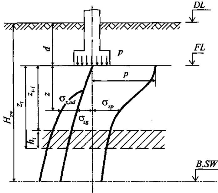
Рисунок Д.6 - Схема до розрахунку підйому основи при набряканні ґрунту
