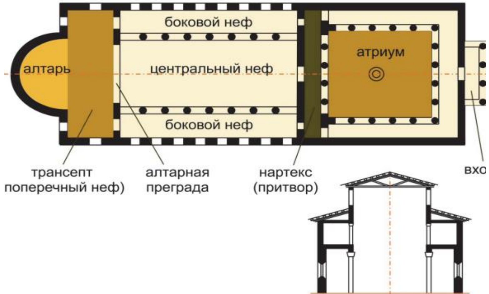
План і конструкція християнської базиліки
