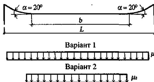
Схема 12. Висячі покриття циліндричної форми
