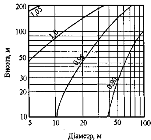
Рисунок 9.5. Коефіцієнт Q для кам'яних будівель і будівель із залізобетонним каркасом
