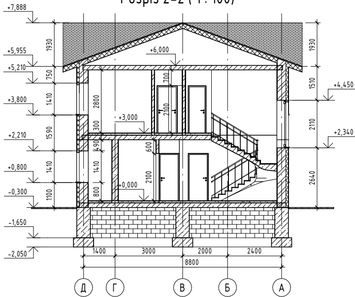
Розріз 2-2 ( 1 : 100)
