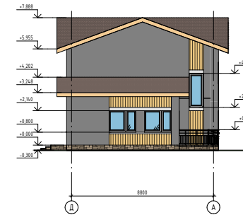
Фасад Д-А (1:100)
