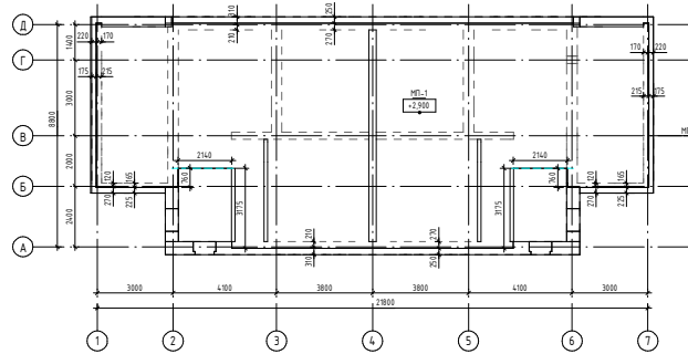
План перекриття (1:100)
