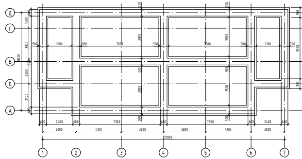
План перекриття (1:100)
