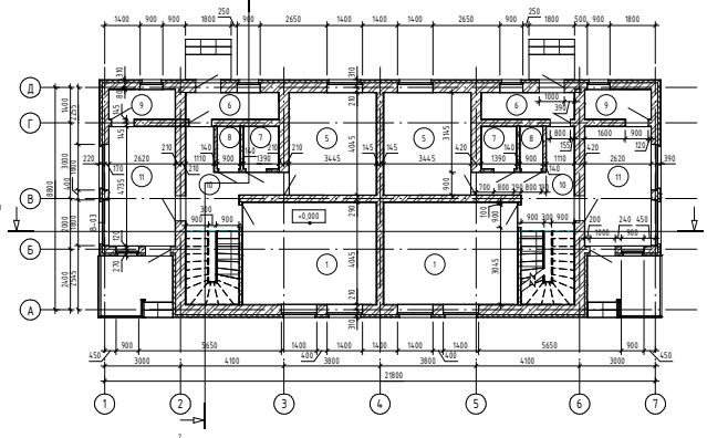
В_АР_ПП_02 Поверх (1:100)
