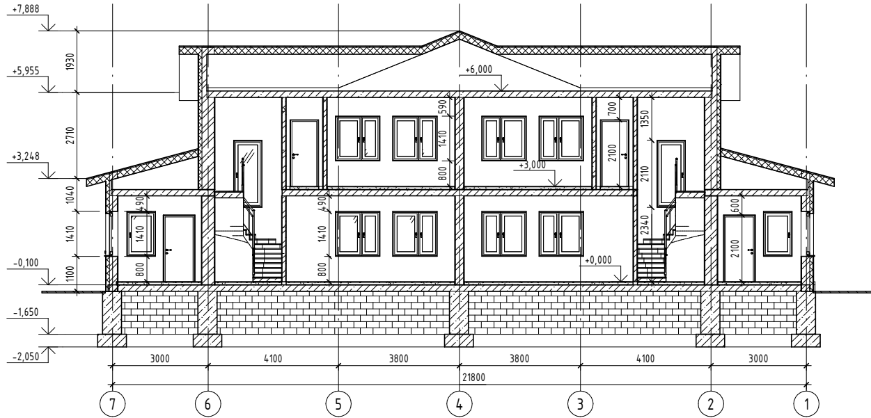
Розріз 2-2 ( 1 : 100)
