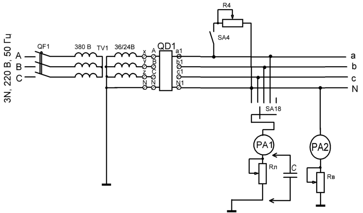
Рис. 1. Схема стенда для дослідження 1-фазного пристрою захисного вимикання
