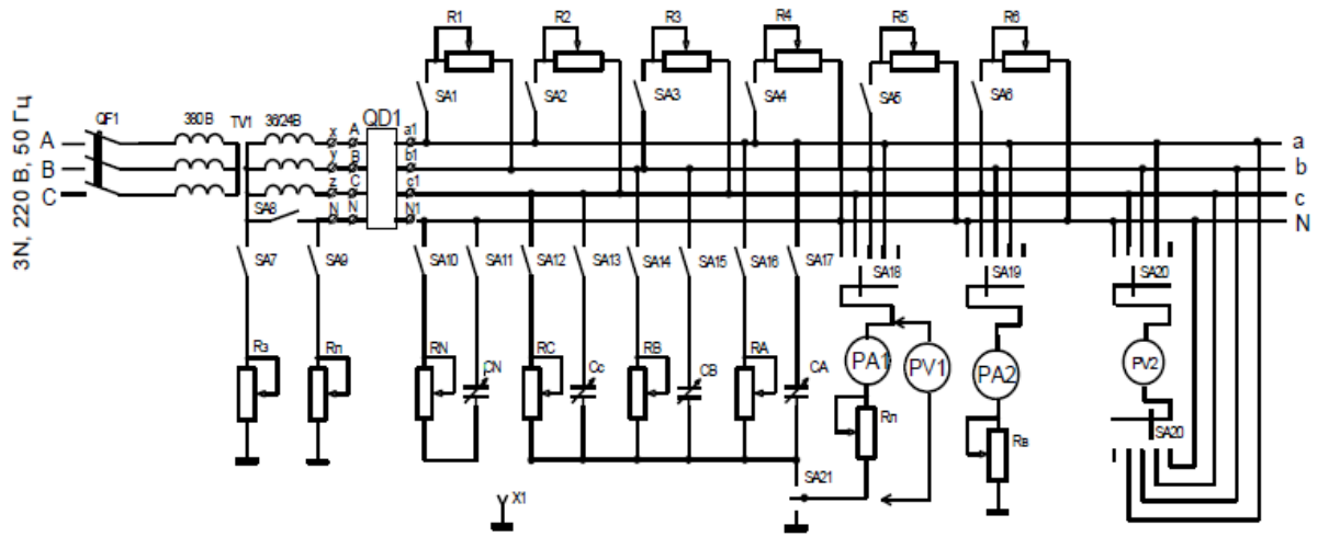
Рис. 2 Схема стенда для дослідження 3-фазного пристрою захисного вимикання
