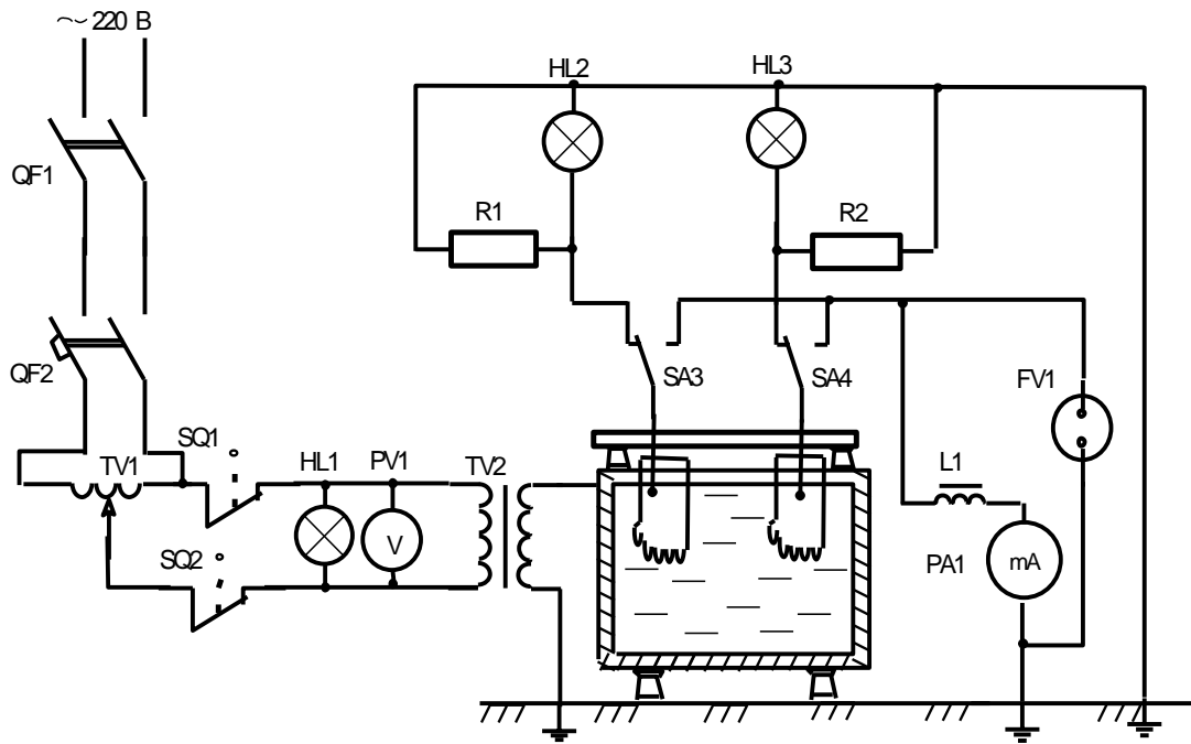
Рис. 1 – Спрощена електрична схема стенда для випробування засобів захисту
