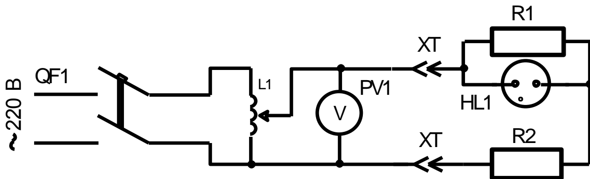
Рис. 2. Схема електрична принципова для перевірки працездатності показників напруги до 1000 В
