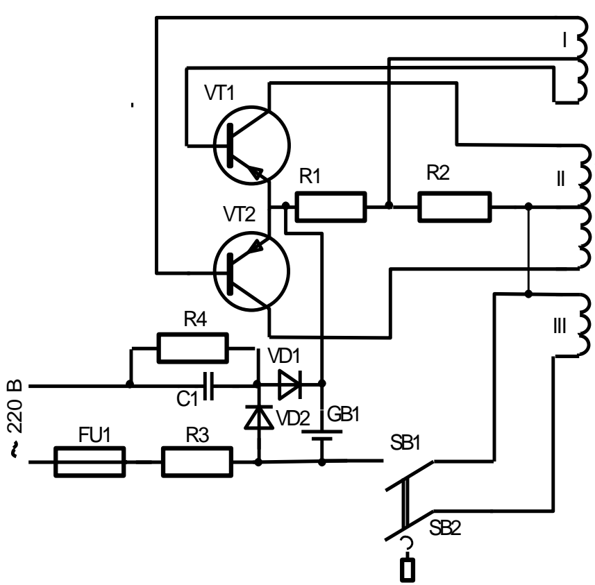
Рис. 3 – Схема електрична принципова пристрою для перевірки працездатності показчика напруги ППУ-2
