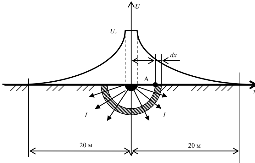
Рис. 5. Розтікання струму в ґрунті через напівсферичний заземлювач
