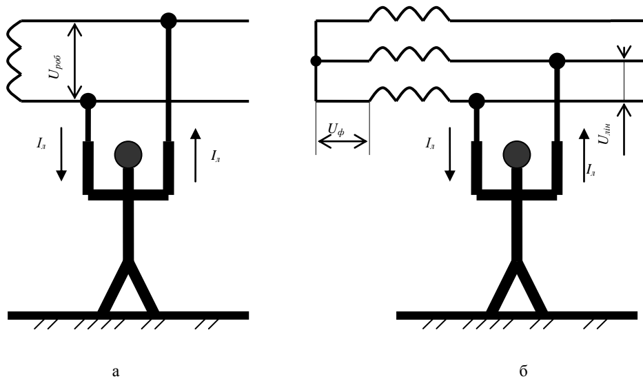
Рис. 2. Схема двофазного доторкання: а – в мережі постійного або однофазного струму; б – в трифазній мережі
