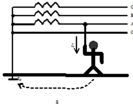
Рис. 2.3. Схема однофазного доторкання при нормальному режимі роботи: а – у трифазній мережі з глухозаземленою нейтраллю;
