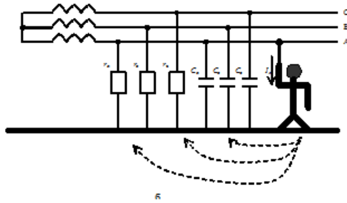
Рис. 3. Схема однофазного доторкання при нормальному режимі роботи:
