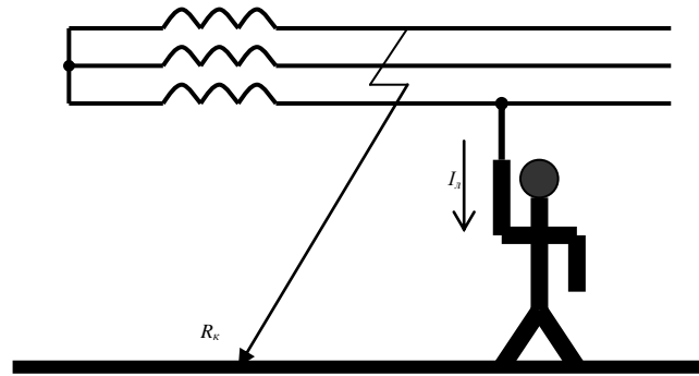
Рис. 4. Схема однофазного доторкання до справної фази несправної електромережі
