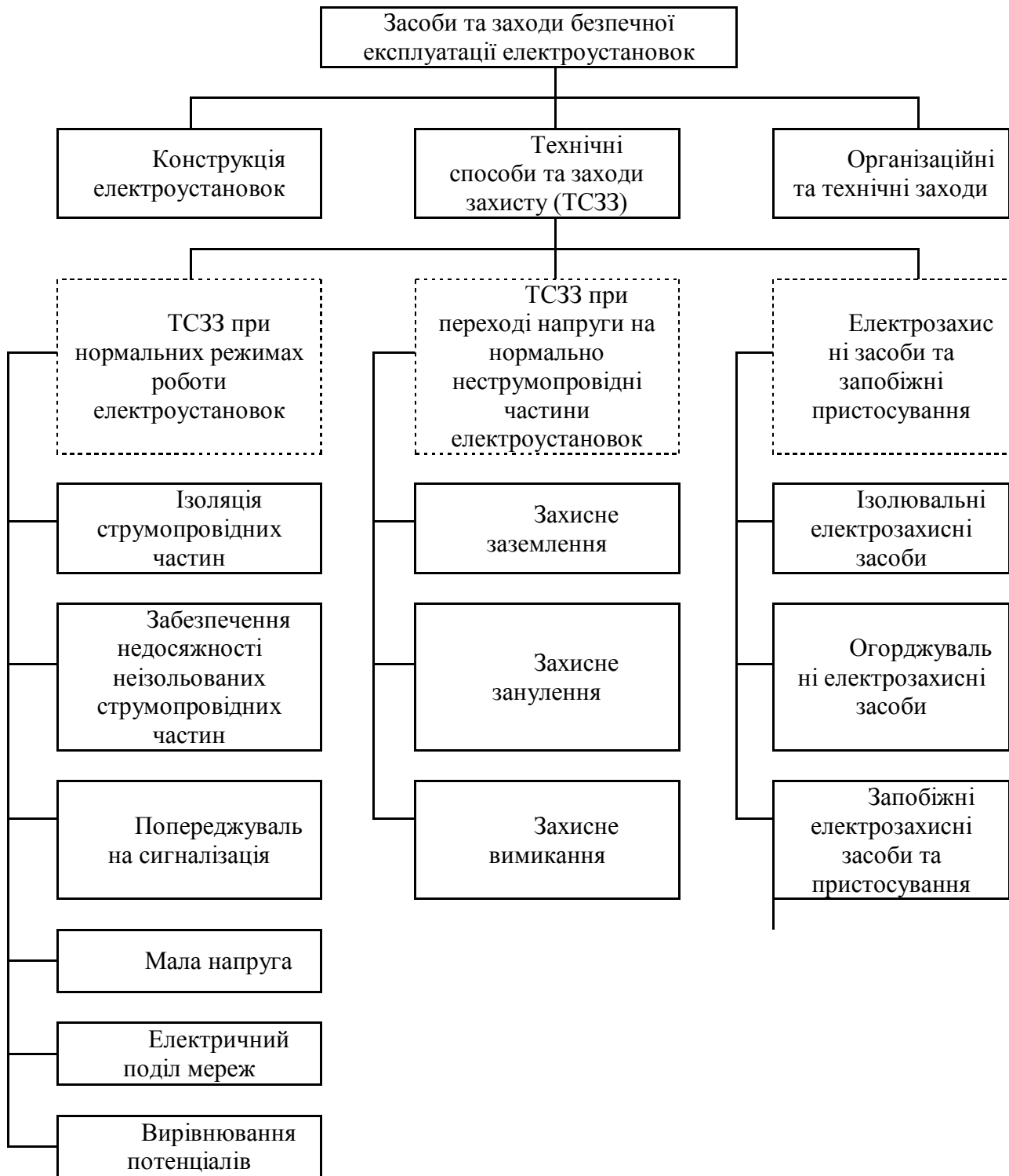
Рис. 8. Класифікація засобів та заходів безпечної експлуатації електроустановок
