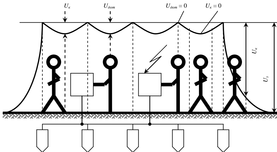
Рис. 1. Вирівнювання потенціалів при контурному заземленні
