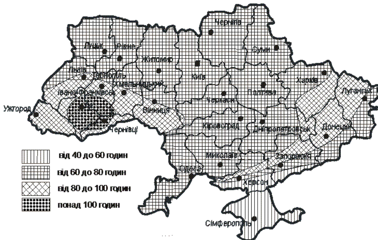
Рис. .1 – Карта середньої тривалості гроз за рік T_{gr} у годинах для території України
