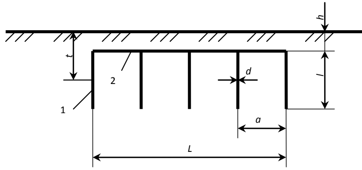
Рис. 2. Схема розташування заземлювачів: 1 – заземлювачі; 2 – заземлювальний провідник
