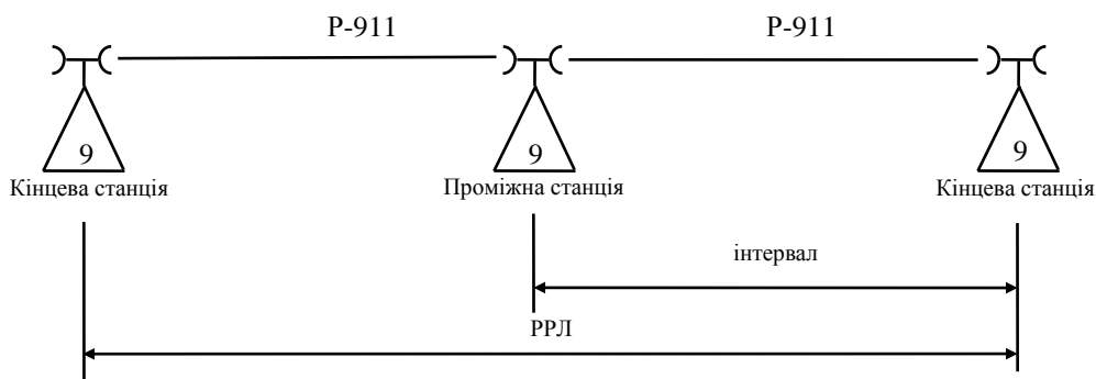
Рис. 13. Радіорелейна лінія
