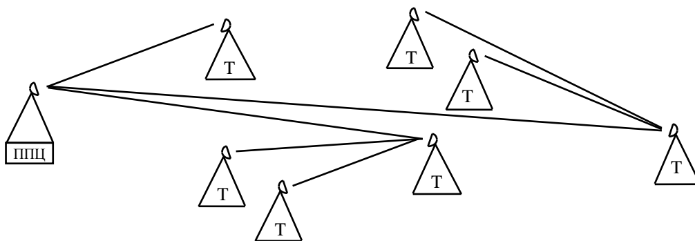
Рис. 10. Радіально-вузловий принцип побудови системи супутникового зв'язку
