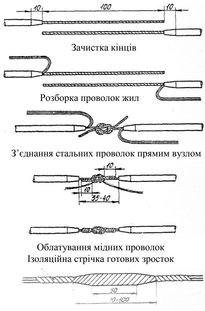
Рис. 44. Зрощування кабелю П-274
