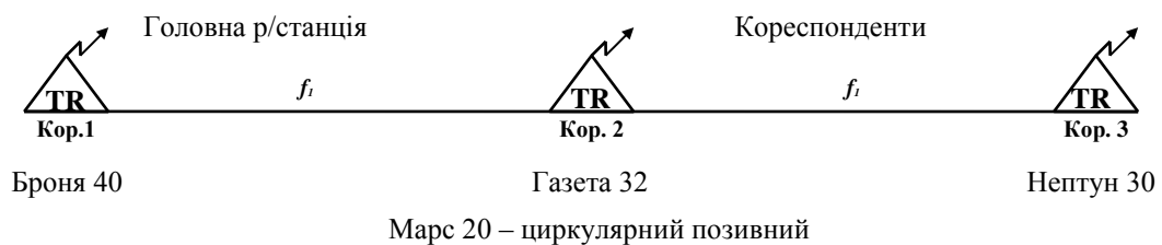
Рис. 32. Радіомережа
