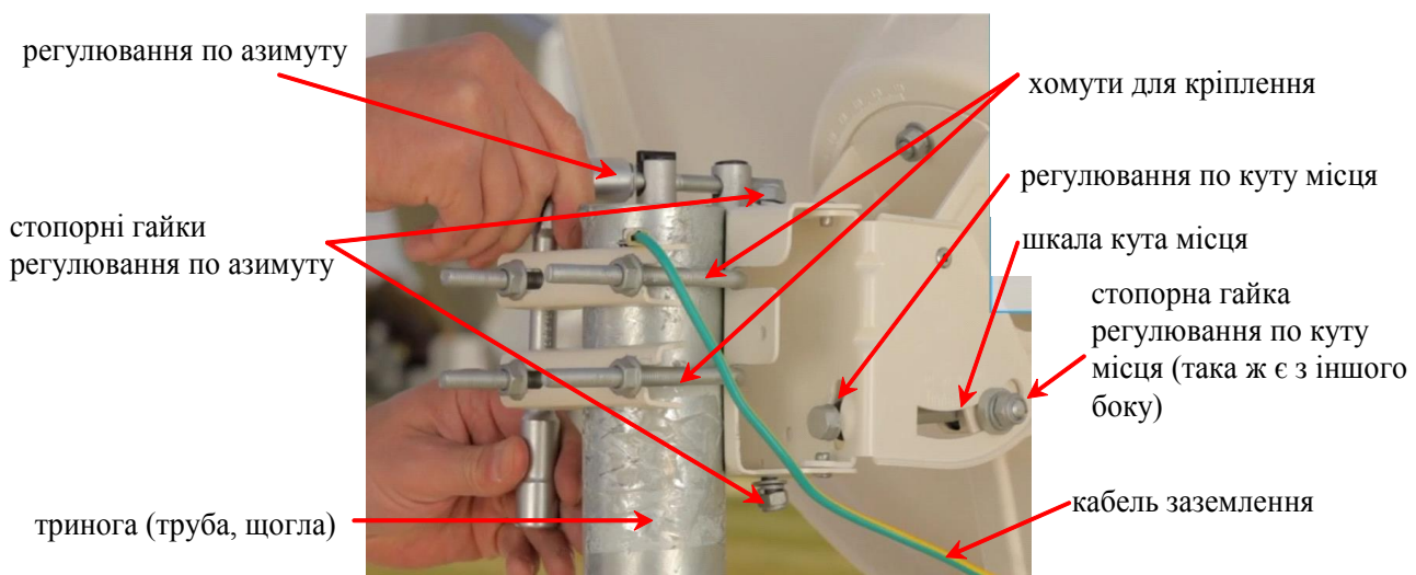
Рис. Д.11.3. Елементи опоро-поворотного пристрою антени
