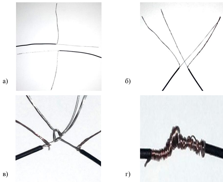
Рис. Д.12.5. Порядок виконання з'єднувальних скруток
