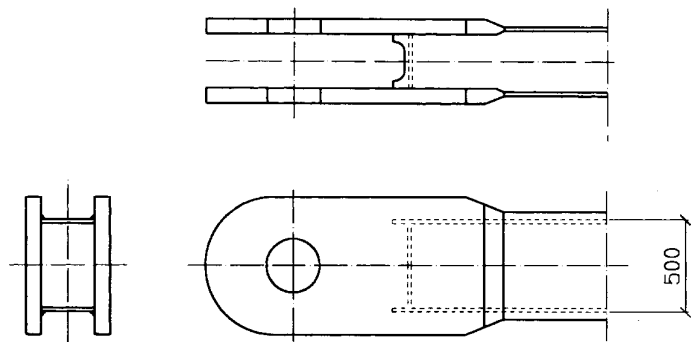
Fig. 7.5.6 Boom-tie construction 3
