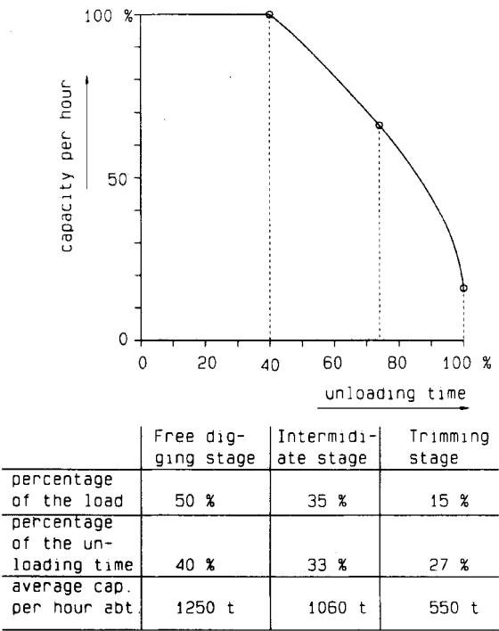
Fig. 1.4.3 Production scheme
