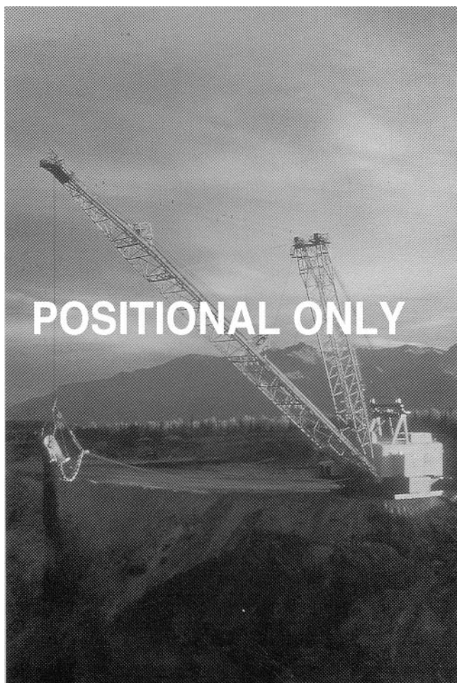
Fig. 9.10.2 Bucyrus-Erie 1300 walking dragline
