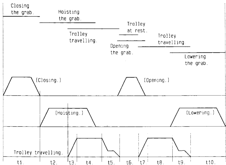
Fig. 3.7.2 Cycle diagram
