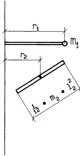
Fig. 3.10.2 Inertia scheme
