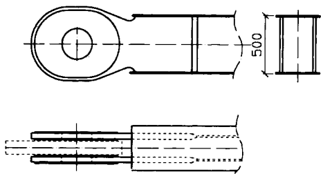
Fig. 7.5.4 Boom-tie construction 1
