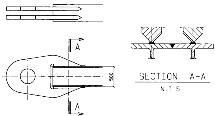
Fig. 7.5.5 Boom-tie construction 2
