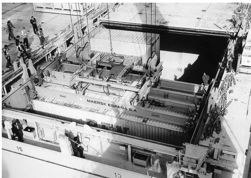
Fig. 6.4.5 Bromma Tandemlift
