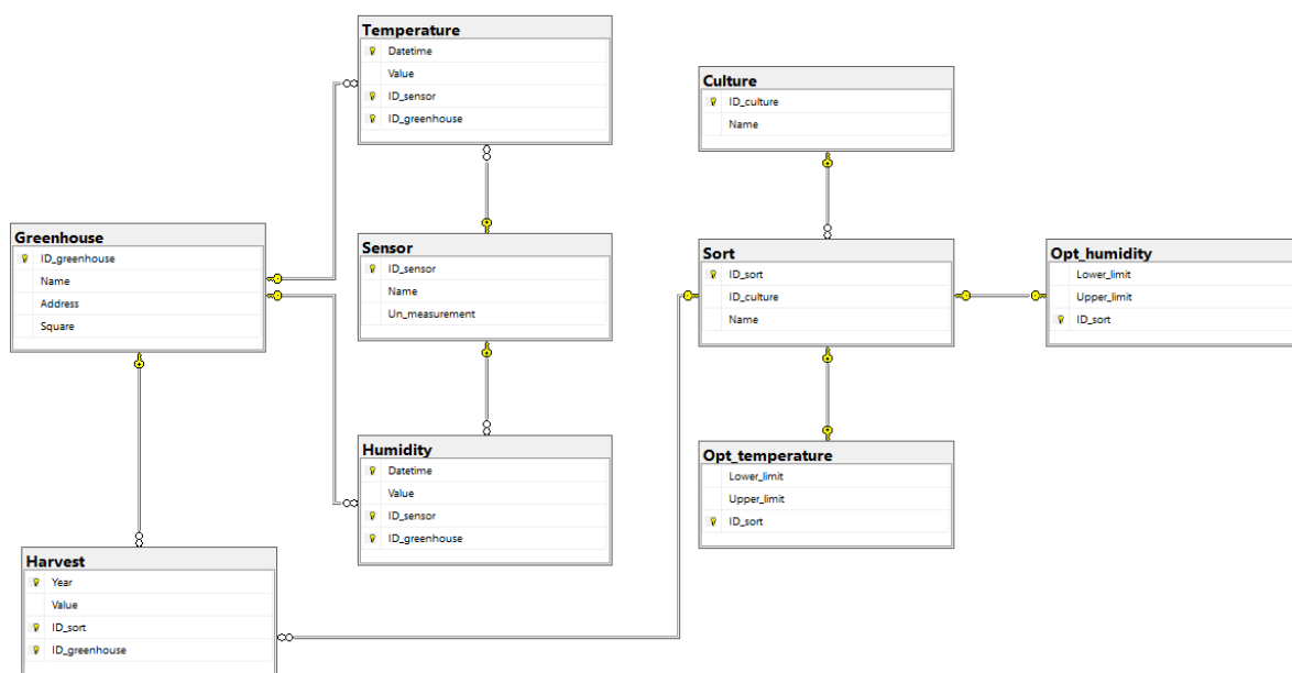
Рис. 3 Схема БД
