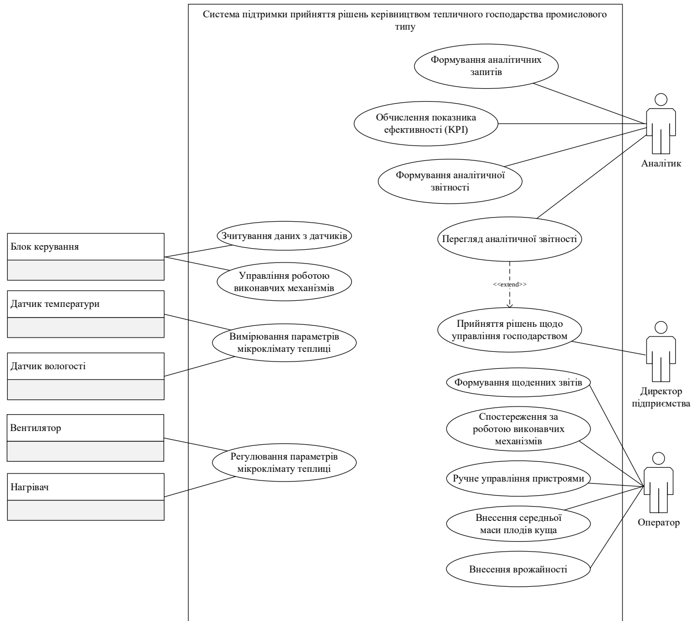
Рис. 1 Діаграма прецедентів
