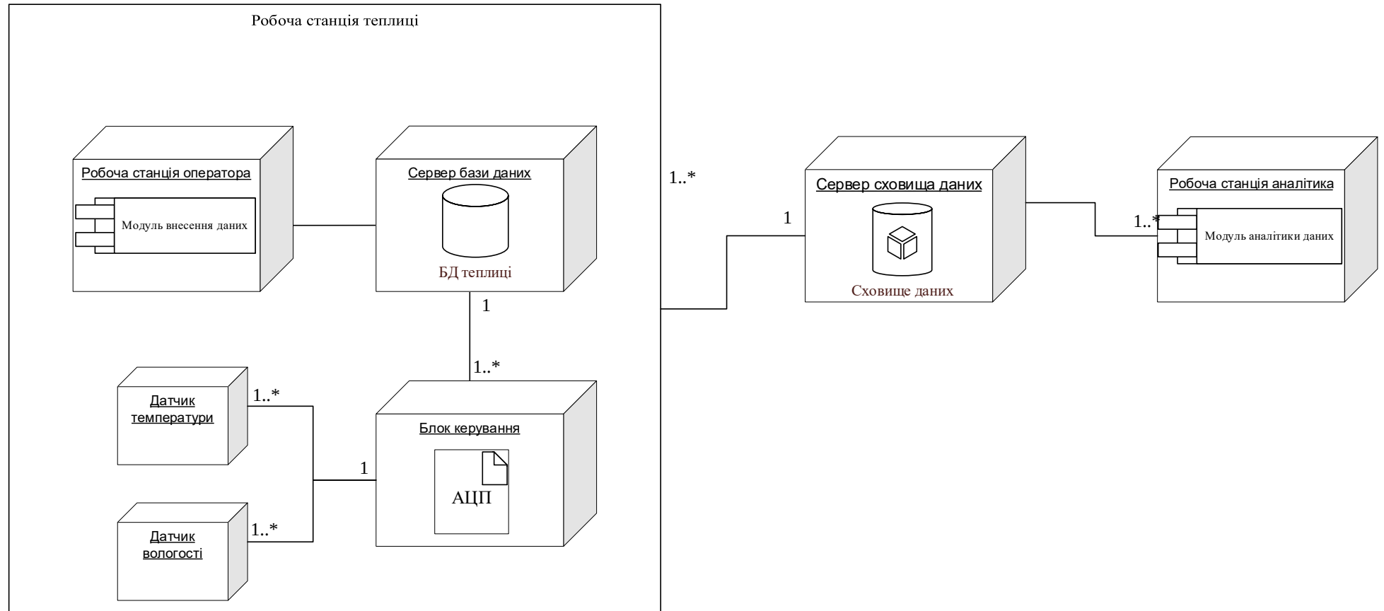
Рис. 2 Діаграма розгортання
