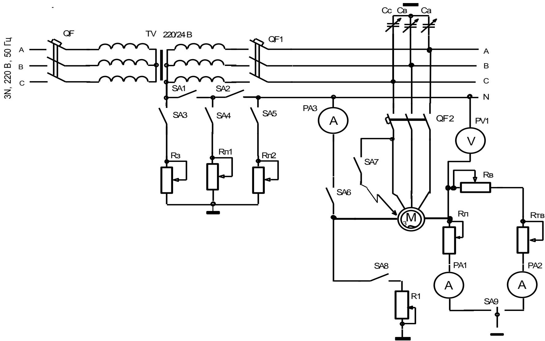
Рис. 2.4. Схема для дослідження ступенів ураження людей та сільськогосподарських тварин електричним струмом
