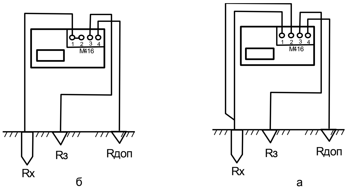
Рис. 3 – Схема вимірювання опору заземлення вимірювачем М-416:
