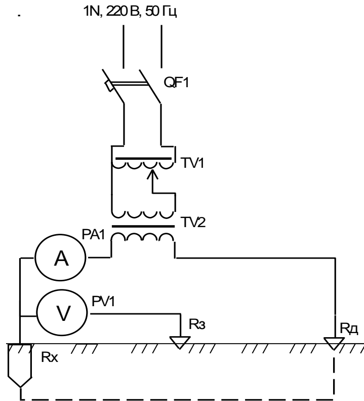
Рис. 1 – Схема вимірювання опору заземлювача методом амперметра-вольтметра
