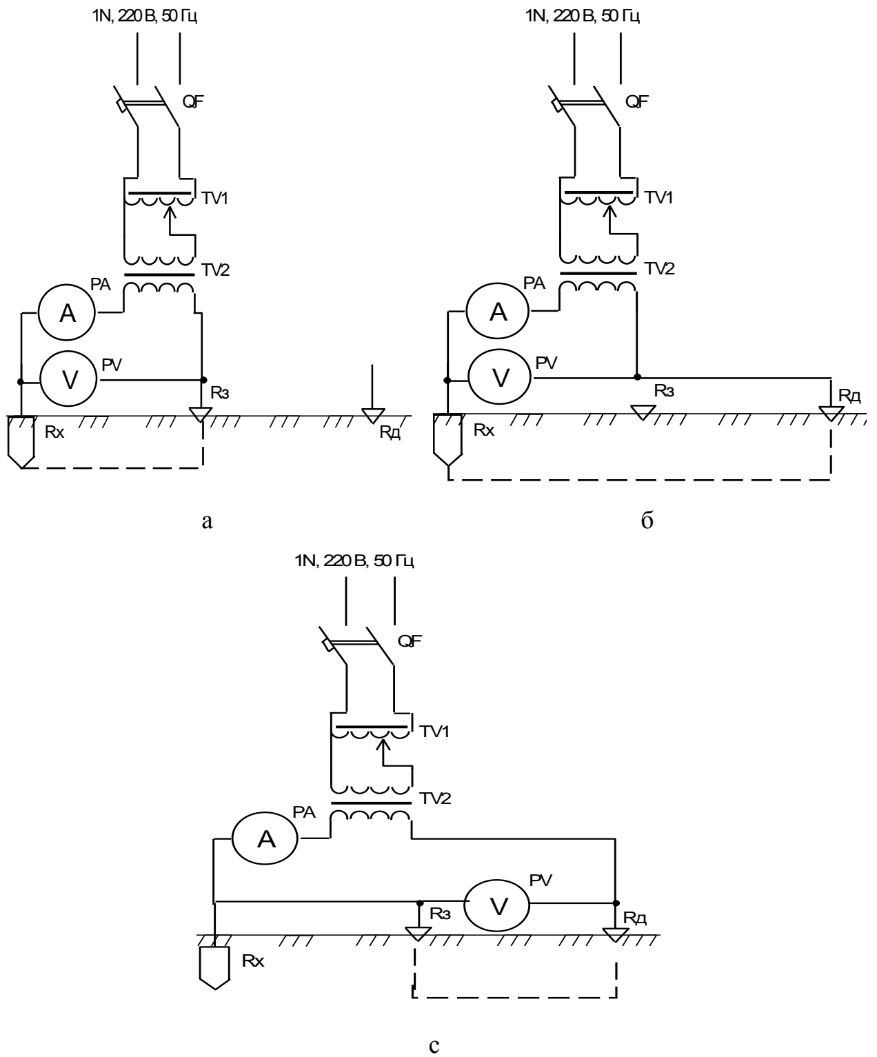
Рис. 2 – Схеми вимірювання опору заземлювача методом ”трьох земель”
