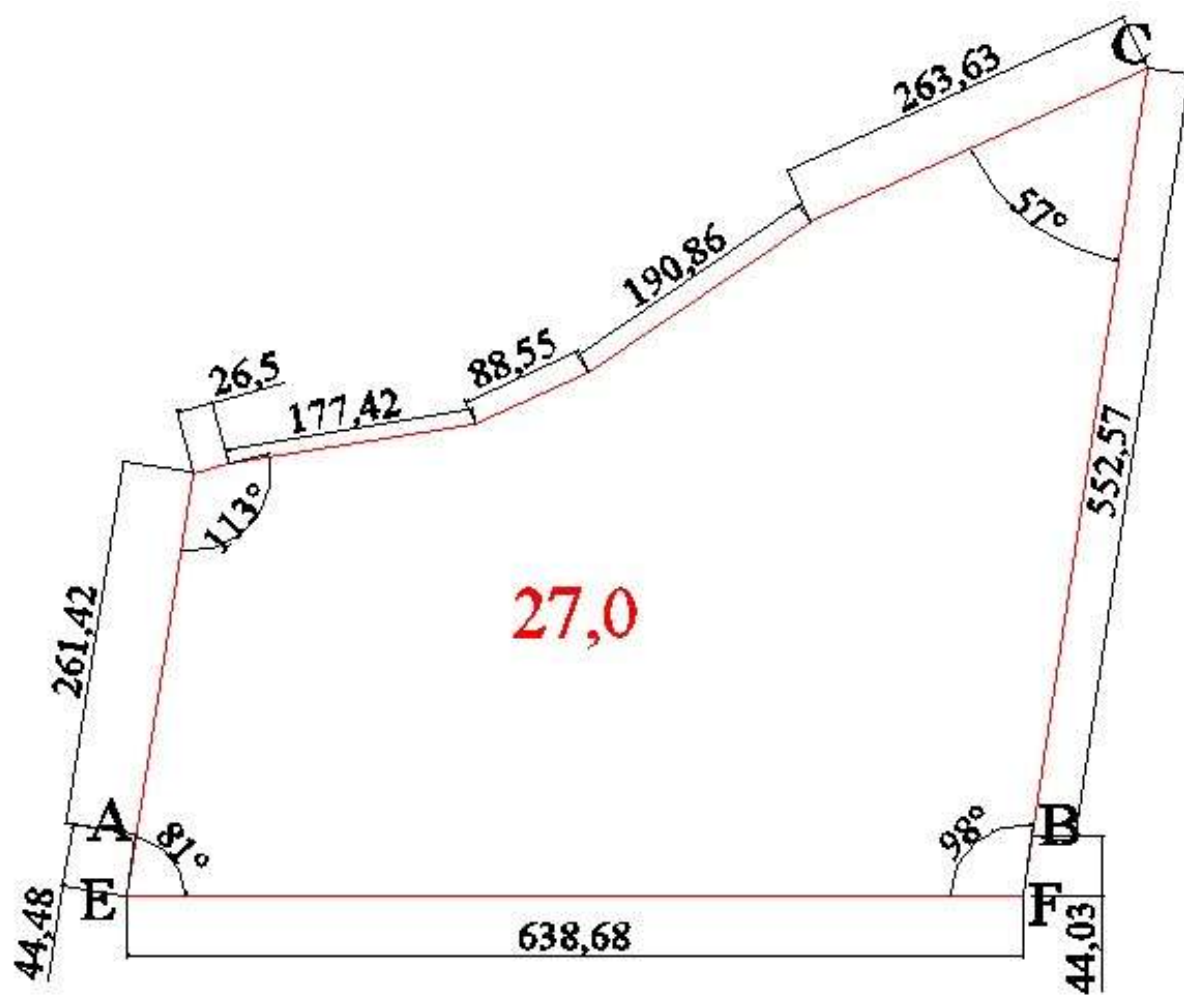
Рис. Абрис виносу в натуру земельної ділянки
